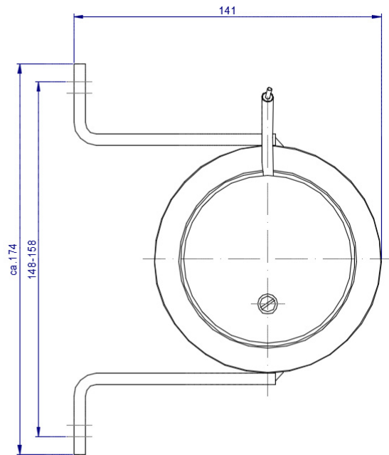
Abmessungen (mm)
